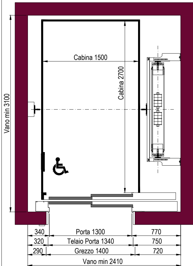
PIANTA VANO CORSA TELAIO PORTE DA 20mm (E1120)
