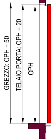
SEZIONE PORTA CON TELAIO DA 20mm (EI120)
