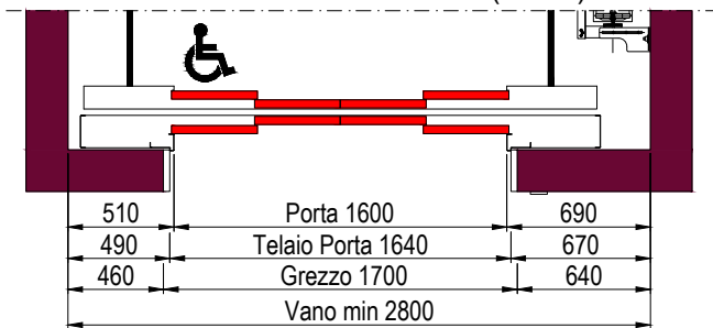
PIANTA VANO CORSA TELAIO PORTE DA 20mm (EI120)
