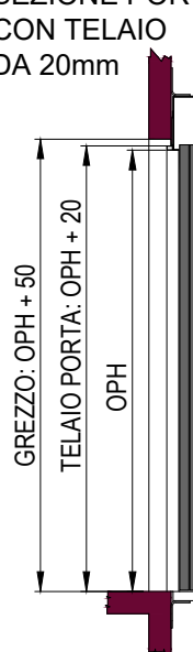
SEZIONE PORTA CON TELAIO DA 20mm (EI120)
