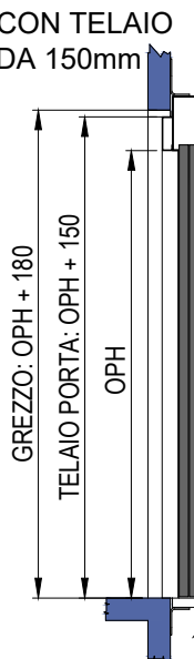
SEZIONE PORTE SENZA TELAIIO (E1120)
