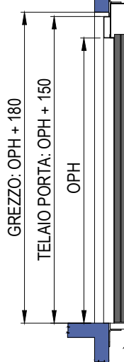
SEZIONE PORTA CON TELAI DA 150mm
