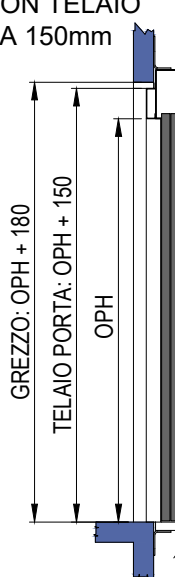
SEZIONE PORTE SENZA TELAIIO (E1120)
