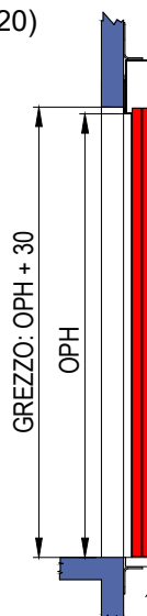
SEZIONE PORTA SENZA TELAIIO (E1120)
