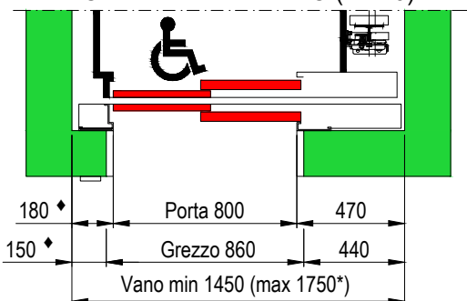
PIANTA VANO CORSA PORTE SENZA TELAIIO (E120)
