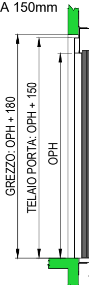
SEZIONE PORTE SENZA TELAIIO (E1120)
