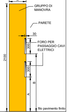
** DETTAGLIO FRONTALE FORI PER PASSAGGIO CAVI ELETTRICI (a cura del Cliente)
