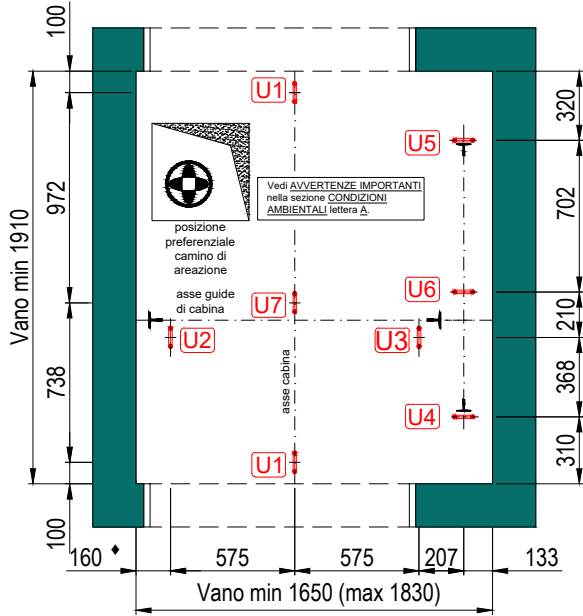
GANCI IN TESTATA (daN) (a cura del Cliente)
