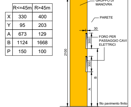
** DETTAGLIO FRONTALE FORI PER PASSAGGIO CAVI ELETTRICI (a cura del Cliente)
