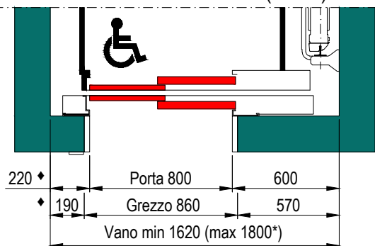
PIANTA VANO CORSA PORTE SENZA TELAIO (EI120)
