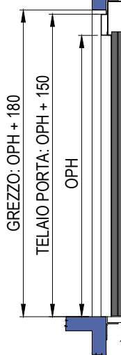
SEZIONE PORTA CON TELAIIO DA 150mm
