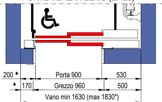
PIANTA VANO CORSA PORTE SENZA TELAIΟ (E1120)
