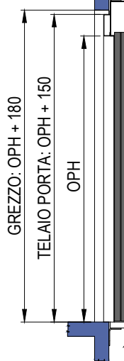
SEZIONE PORTA CON TELAIΟ DA 150mm
