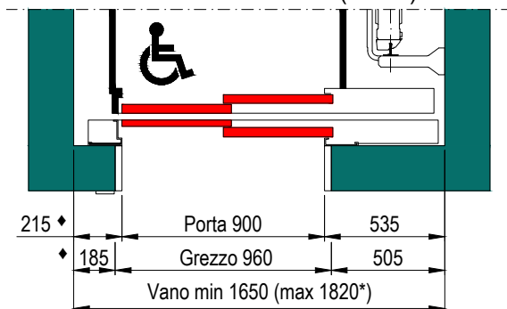
PIANTA VANO CORSA PORTE SENZA TELAIIO (E1120)
