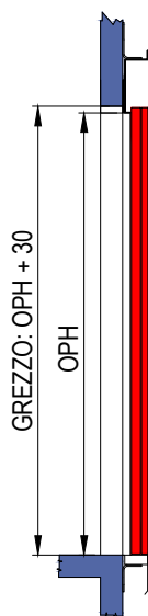
SEZIONE PORTA SENZA TELAIO (E1120)
