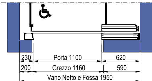
PIANTA VANO CORSA PORTE SENZA STIPITI - E1120
