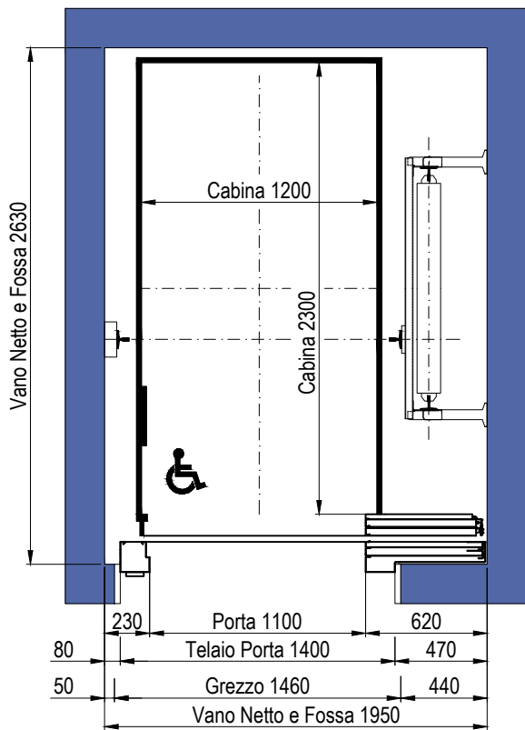
PIANTA VANO CORSA PORTE CON TELAIO DA 150mm
