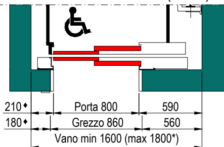
PIANTA VANO CORSA PORTE SENZA TELAIO (EI120)
