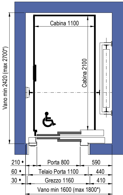
PIANTA VANO CORSA TELAIO PORTE DA 150mm
