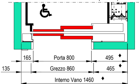
PIANTA VANO CORSA PORTE SENZA TELAIO (EI120)
