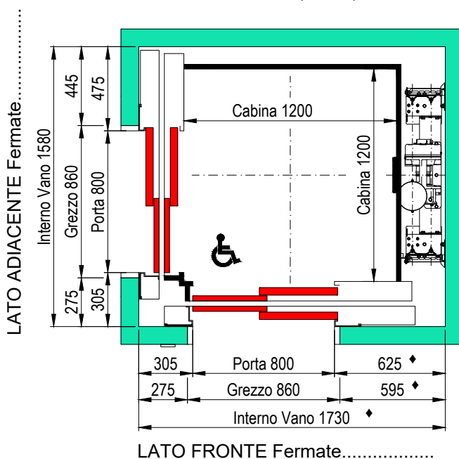
PIANTA VANO CORSA PORTE SENZA TELAIIO (E1120)
