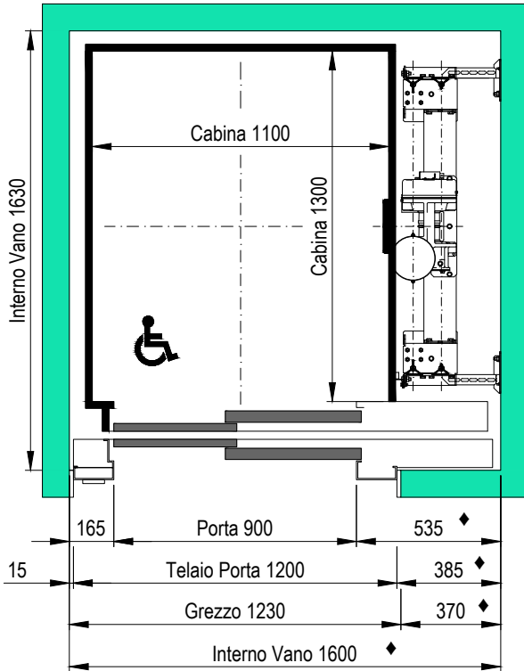
PIANTA VANO CORSA TELAIO PORTE DA 150mm
