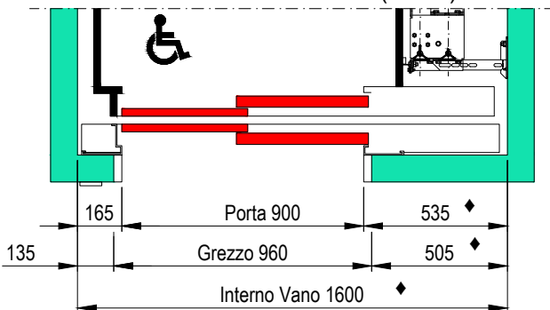
PIANTA VANO CORSA PORTE SENZA TELAIO (EI120)
