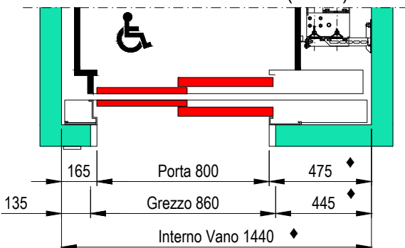
PIANTA VANO CORSA PORTE SENZA TELAIIO (E120)
