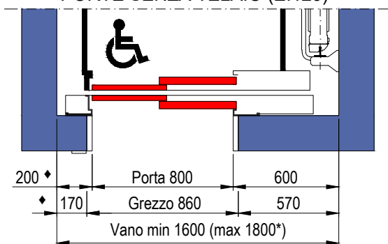
PIANTA VANO CORSA PORTE SENZA TELAIO (E1120)
