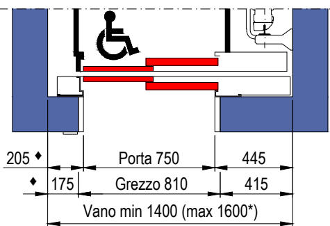
PIANTA VANO CORSA PORTE SENZA TELAIO (E120)
