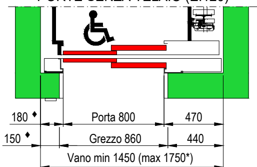
PIANTA VANO CORSA PORTE SENZA TELAIIO (E1120)
