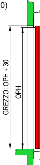
SEZIONE PORTA SENZA TELAIIO (E1120)
