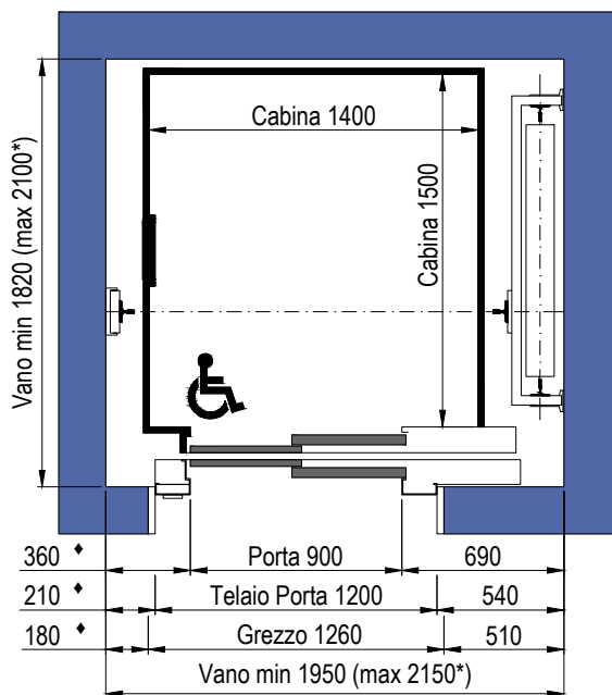
PIANTA VANO CORSA TELAIO PORTE DA 150mm
