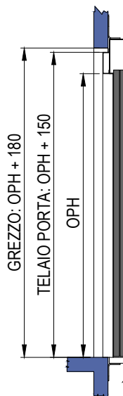
SEZIONE PORTA CON TELAIO DA 150mm
