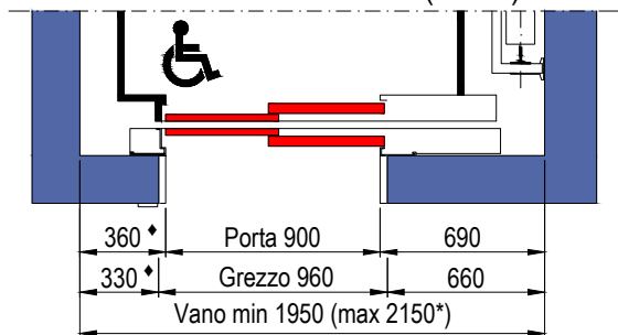
PIANTA VANO CORSA PORTE SENZA TELAIO (EI120)
