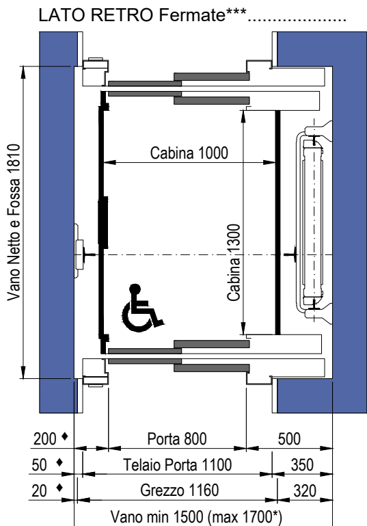
PIANTA VANO CORSA TELAIO PORTE DA 150mm
