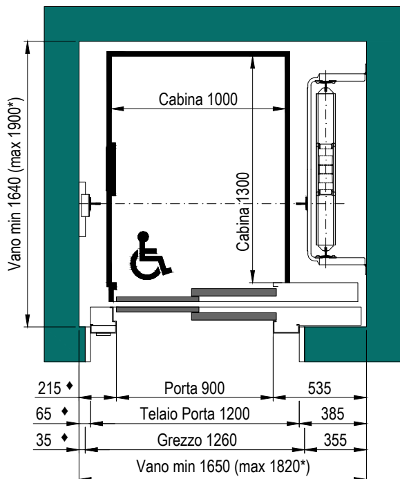
PIANTA VANO CORSA TELAIO PORTE DA 150mm
