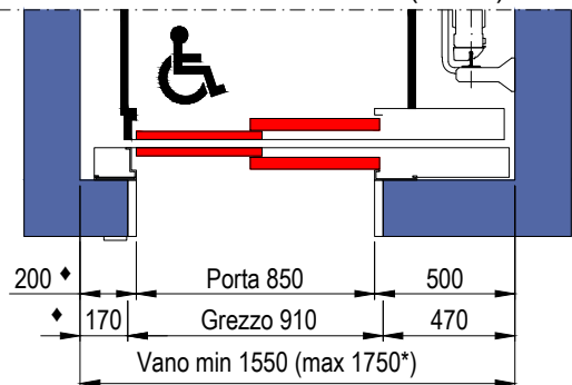
PIANTA VANO CORSA PORTE SENZA TELAIIO (EI120)
