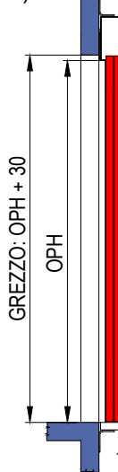
SEZIONE PORTE SENZA TELAIIO (EI120)
