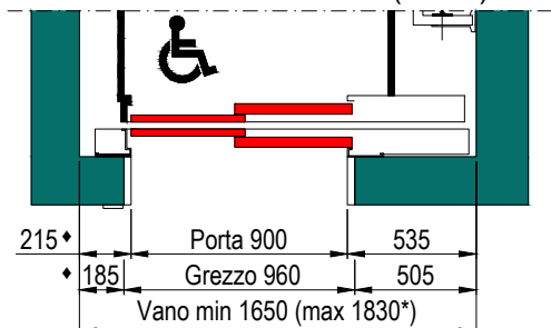
PIANTA VANO CORSA PORTE SENZA TELAIO (EI120)
