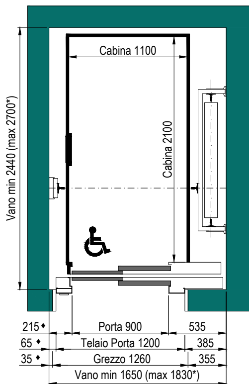
PIANTA VANO CORSA TELAIO PORTE DA 150mm
