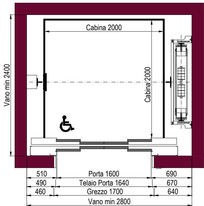
PIANTA VANO CORSA TELAIO PORTE DA 20mm
