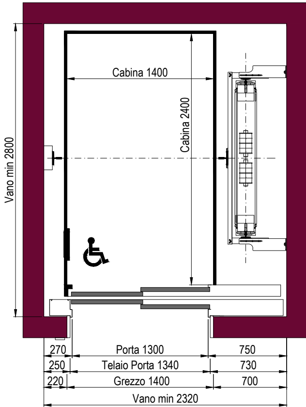
PIANTA VANO CORSA TELAIO PORTE DA 20mm
