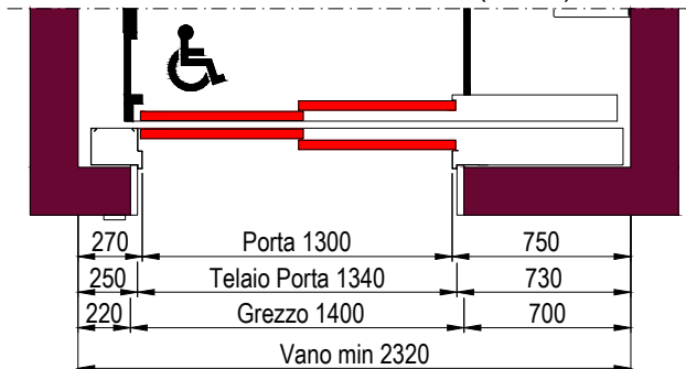
PIANTA VANO CORSA TELAIO PORTE DA 20mm (E1120)
