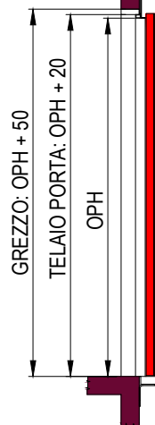
SEZIONE PORTA CON TELAIIO DA 20mm (E1120)
