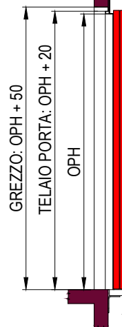
SEZIONE PORTA CON TELAIIO DA 20mm (EI120)
