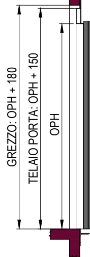
SEZIONE PORTA CON TELAIIO DA 20mm (EI120)
