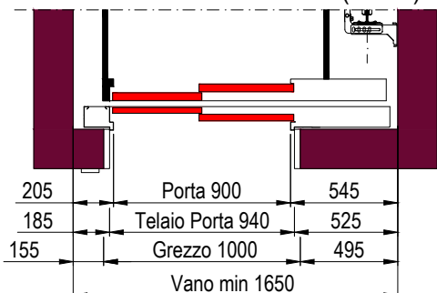
PIANTA VANO CORSA TELAIO PORTE DA 20mm (EI120)
