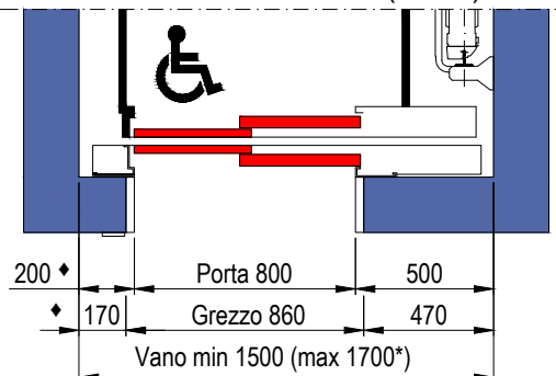
PIANTA VANO CORSA PORTE SENZA TELAI (E1120)
