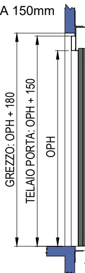
SEZIONE PORTA CON TELAI DA 150mm
