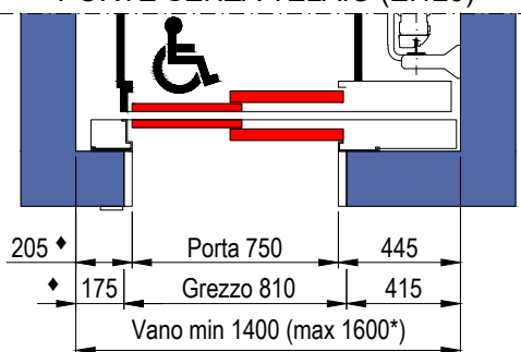
PIANTA VANO CORSA PORTE SENZA TELAIIO (E1120)
