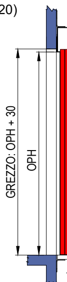
SEZIONE PORTE SENZA TELAIIO (E1120)
