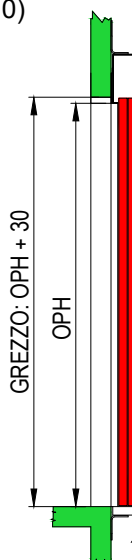
SEZIONE PORTE SENZA TELAIIO (EI120)
