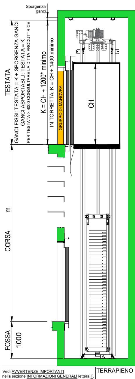
SEZIONE VANO CORSA
