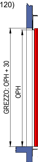
SEZIONE PORTA SENZA TELAIO (EI120)
