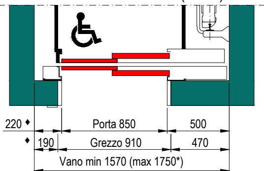
PIANTA VANO CORSA PORTE SENZA TELAIO (EI120)
