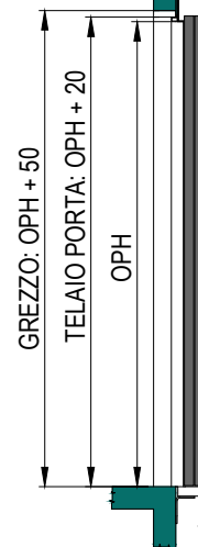
SEZIONE PORTA CON TELAIO DA 90mm (EI60 - EI120)
