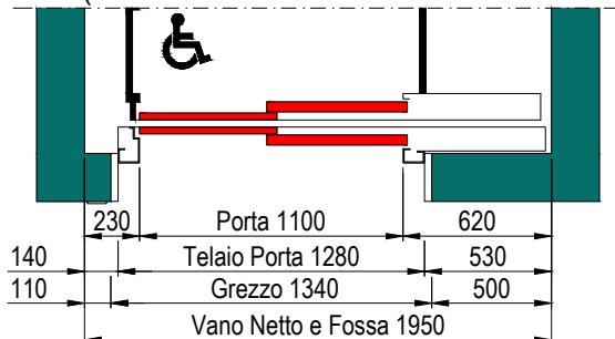
PIANTA VANO CORSA TELAIO PORTE DA 90mm - EI60-120 (Prodotto da richiedere in deviazione)
