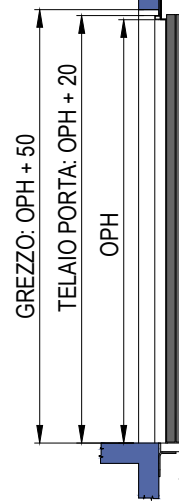
SEZIONE PORTA CON TELAIO DA 90mm (EI60 - EI120)
