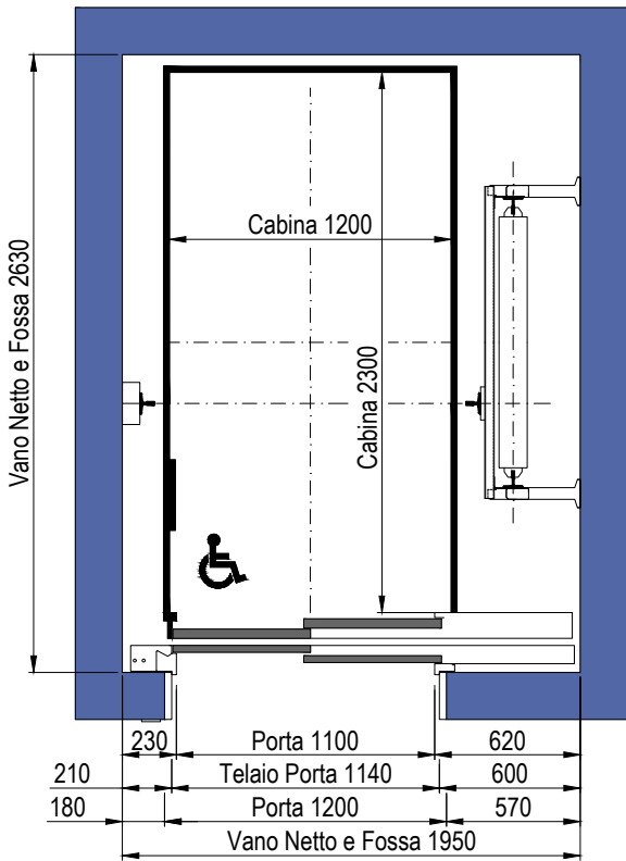
PIANTA VANO CORSA TELAIO PORTE DA 20mm
