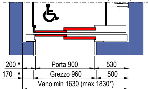
PIANTA VANO CORSA PORTE SENZA TELAIO (EI120)
