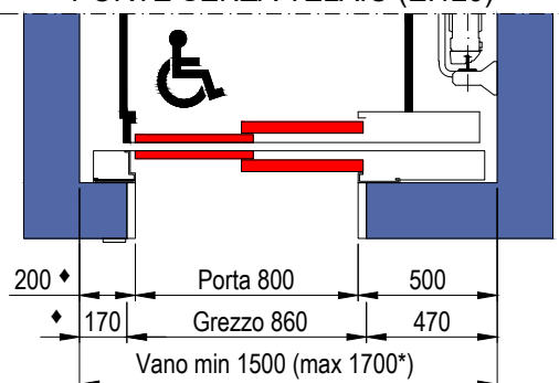
PIANTA VANO CORSA PORTE SENZA TELAIO (E1120)
