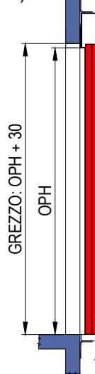
SEZIONE PORTE SENZA TELAIO (E1120)
