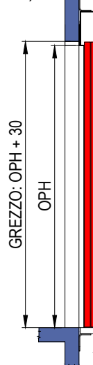
SEZIONE PORTE SENZA TELAIIO (EI120)
