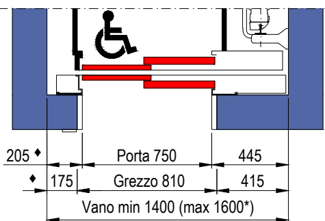
PIANTA VANO CORSA PORTE SENZA TELAIIO (EI120)
