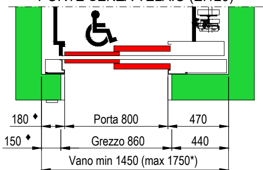
PIANTA VANO CORSA PORTE SENZA TELAIIO (EI120)
